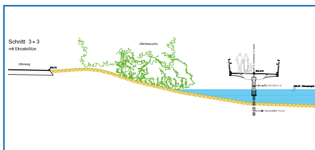
Schnitt durch die Stegkonstruktion aus Stahl mit Einzelstütze
